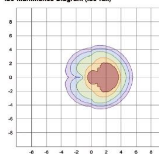
Iso-Illuminance Diagram (Iso-lux)
