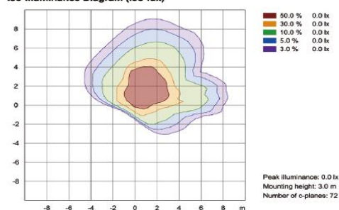
Iso-illuminance Diagram (Iso-lux)
