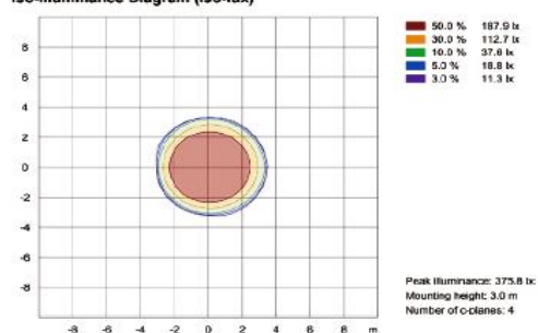
Iso-illuminance Diagram (Iso-lux)
