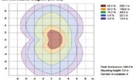
Iso-Illuminance Diagram (iso-lux)
