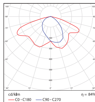
Puissance: 100.0 W
