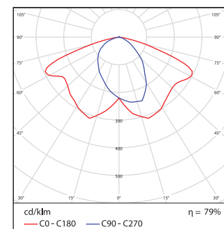
Puissance: 250.0 W
